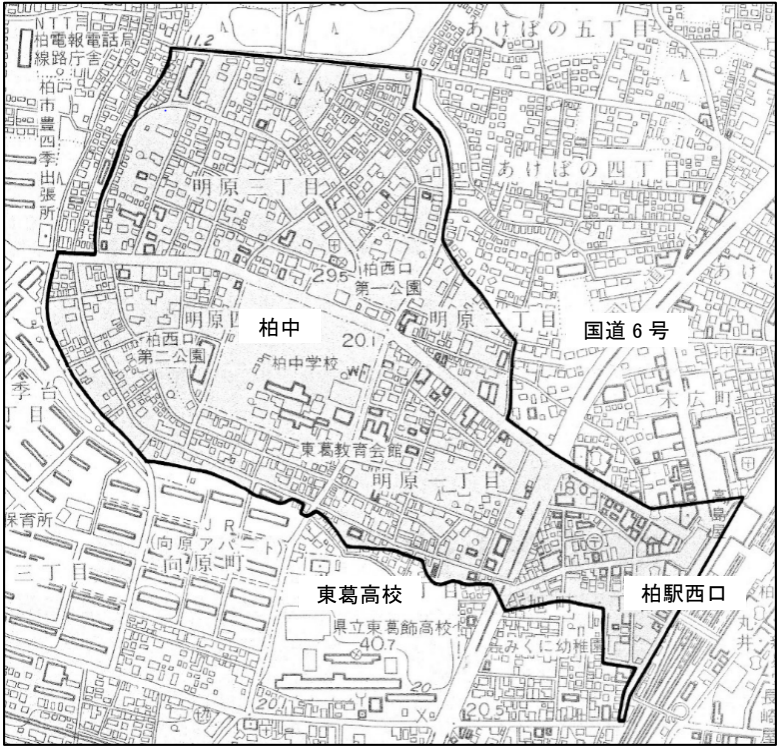
図 4-3-1 柏駅西口区画整理事業の範囲
